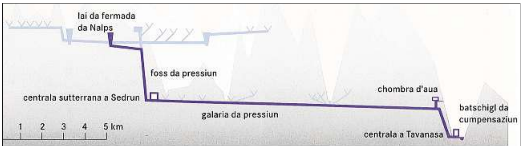
Dissegn simplifitgà d'ina ovra d'accumulaziun idroelectrica en Surselva.
