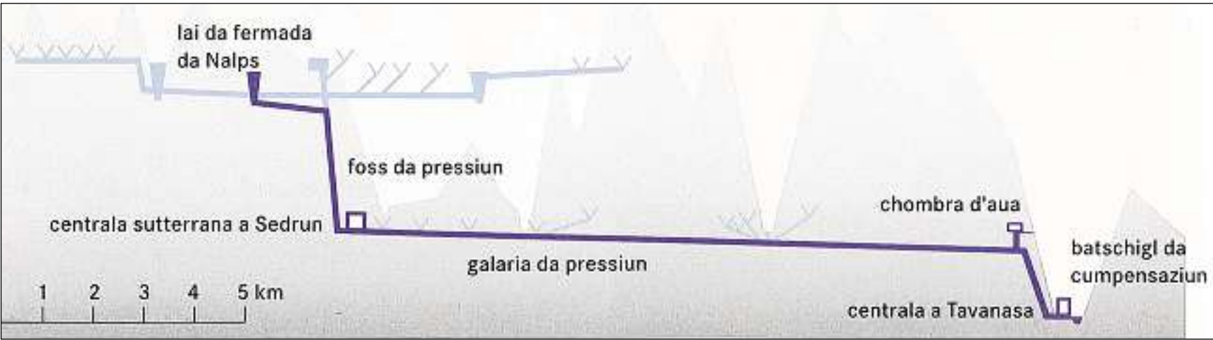
Disegn simplifitgà d'ina ovra d'accumulaziun idroelectrica en Surselva.
